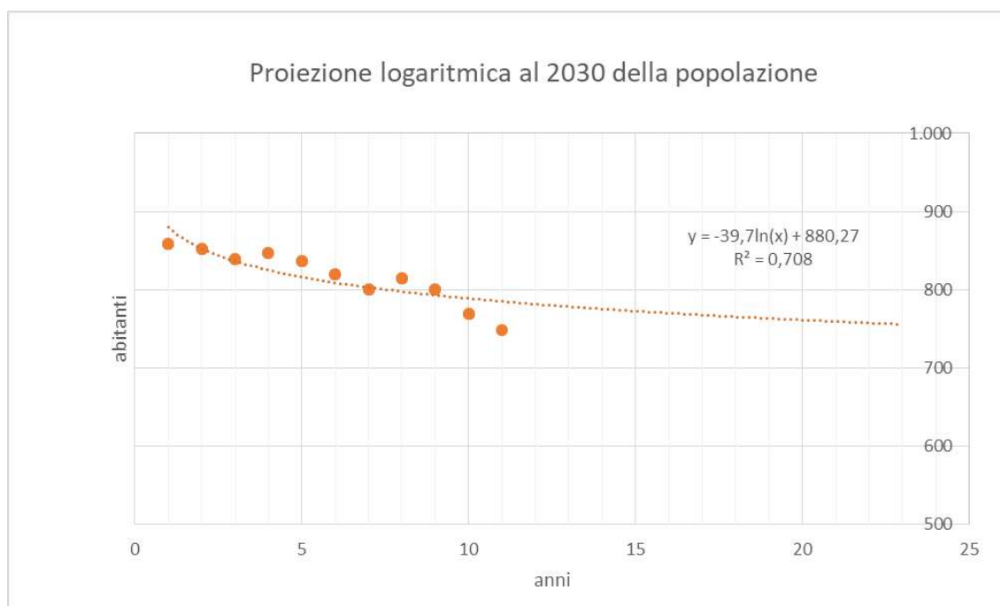
Figura 39 - Grafico di dispersione della popolazione di Sant'Angelo All'Esca nel decennio 2010/2019 con rappresentazione della linea di tendenza di tipo logaritmico al 2030
