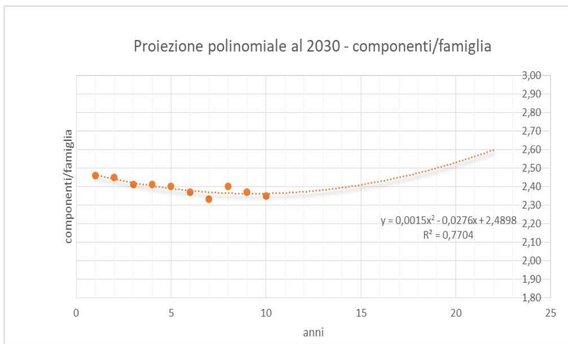
Figura 45- Grafico di dispersione del numero di componenti/famiglia di Sant'Angelo All'Esca nel decennio 2010/2019 con rappresentazione della linea di tendenza di tipo polinomiale al 2030
