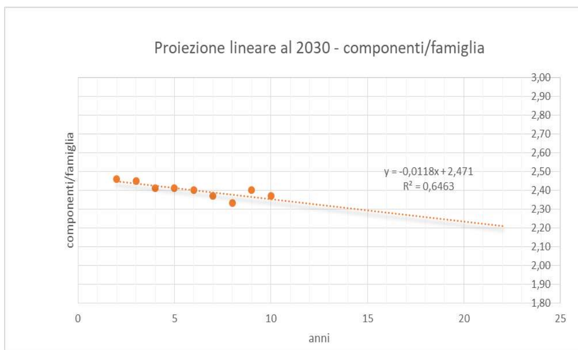
Figura 43- Grafico di dispersione del numero di componenti/famiglia di Sant'Angelo All'Esca nel decennio 2010/2019 con rappresentazione della linea di tendenza di tipo lineare al 2030
