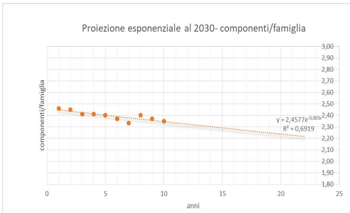
Figura 47- Grafico di dispersione del numero di componenti/famiglia di Sant'Angelo All'Esca nel decennio 2009/2019 con rappresentazione della linea di tendenza di tipo esponenziale al 2030
