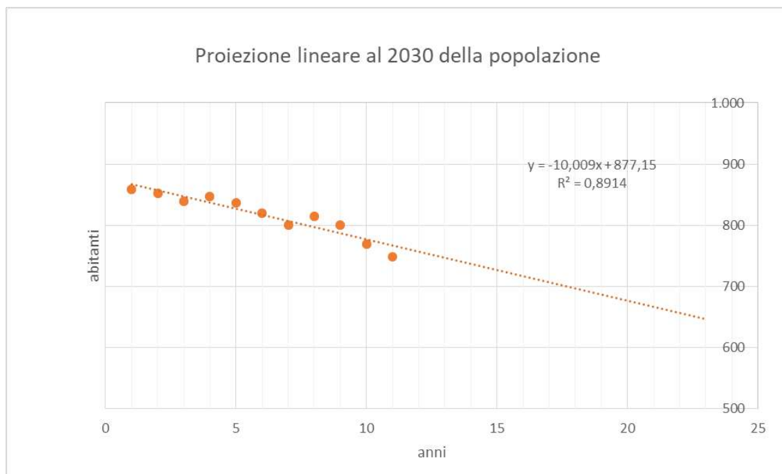
Figura 38 - Grafico di dispersione della popolazione di Sant'Angelo All'Esca nel decennio 2010/2019 con rappresentazione della linea di tendenza di tipo lineare al 2030
