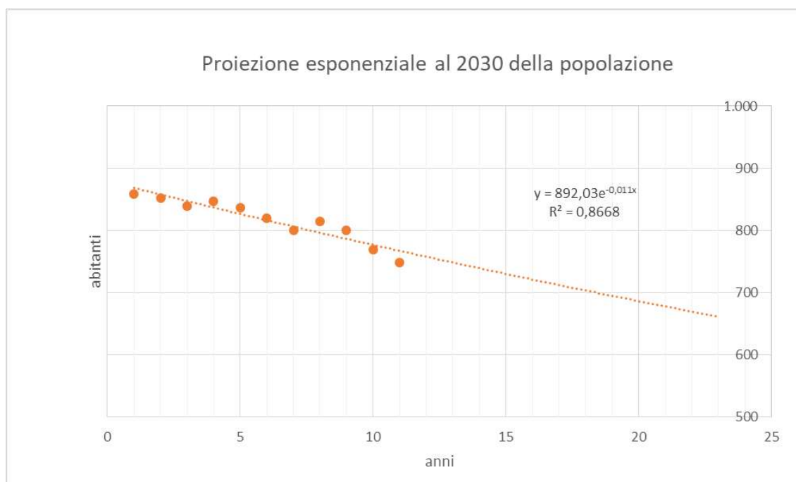
Figura 42- Grafico di dispersione della popolazione di Sant'Angelo All'Esca nel decennio 2010/2019 con rappresentazione della linea di tendenza di tipo esponenziale al 2030
