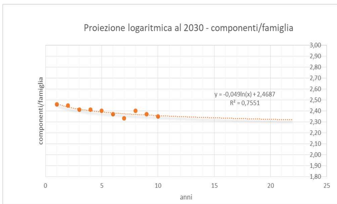
Figura 44- Grafico di dispersione del numero di componenti/famiglia di Sant'Angelo All'Esca nel decennio 2010/2020 con rappresentazione della linea di tendenza di tipo logaritmico al 2030
