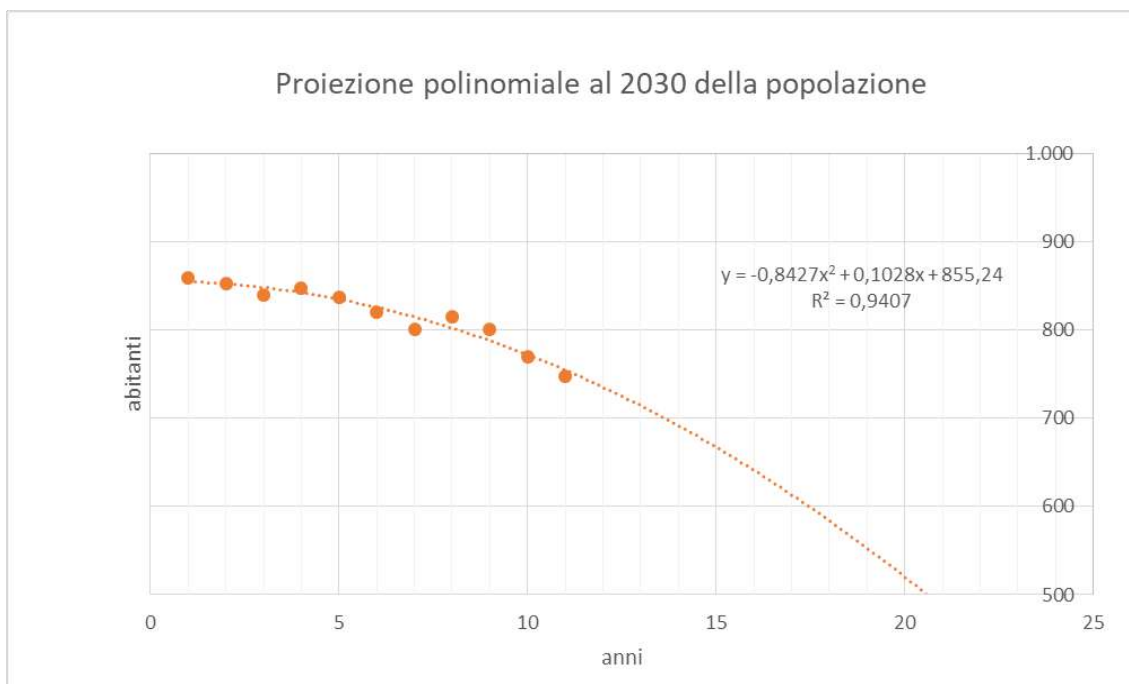
Figura 40- Grafico di dispersione della popolazione di Sant'Angelo All'Esca nel decennio 2010/2019 con rappresentazione della linea di tendenza di tipo polinomiale al 2030
