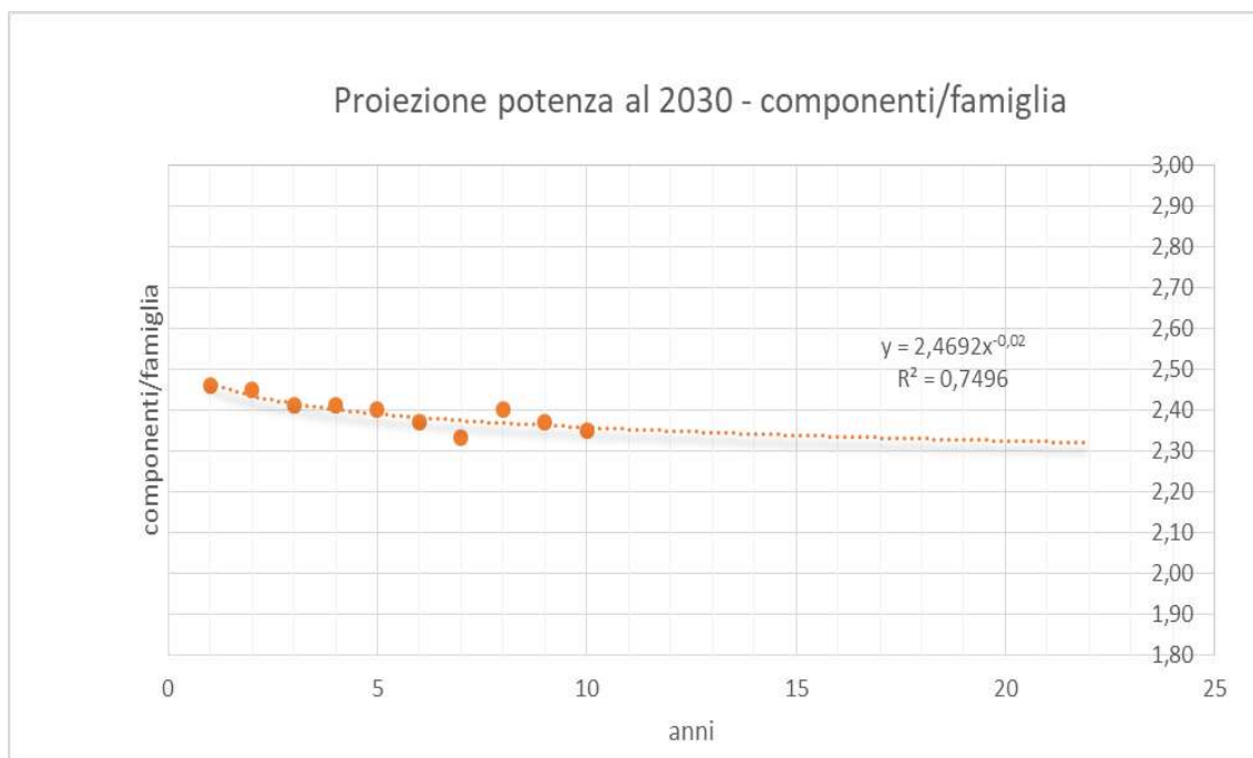
Figura 46- Grafico di dispersione del numero di componenti/famiglia di Sant'Angelo All'Esca nel decennio 2010/2019 con rappresentazione della linea di tendenza di tipo di potenza al 2030
